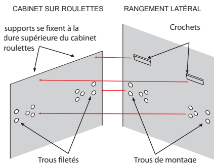
COFFRE SUPÉRIEUR AVEC TROUS FILETÉS
