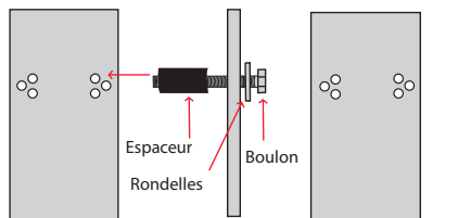
Vue latérale de l'armoire latérale
